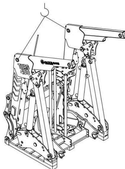
Рисунок 31 – Схема строповки
