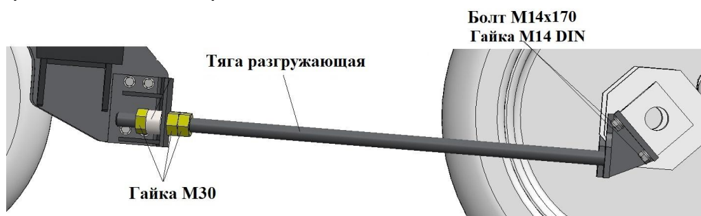
Рисунок 8 – Тяга опорная
