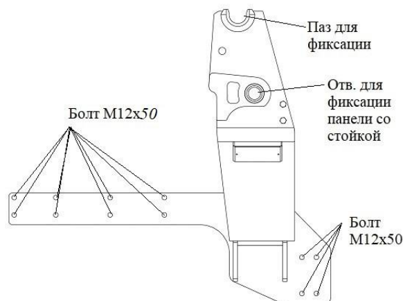
Рисунок 5 – Панель левая
