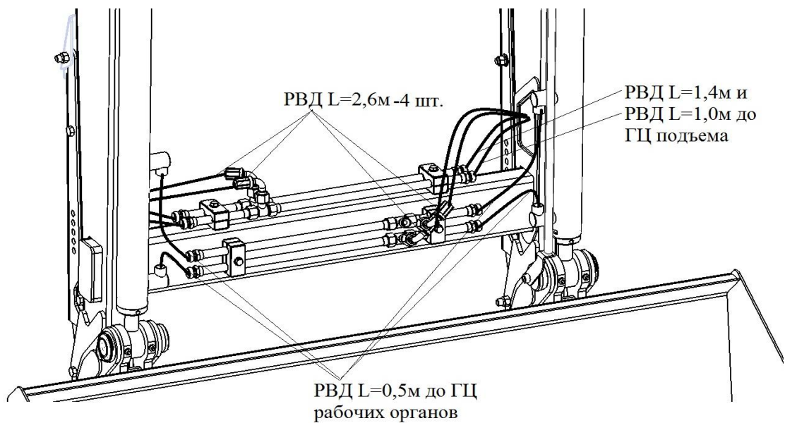
Рисунок 16 – Подсоединение гидросистемы погрузчика к гидросистеме трактора
