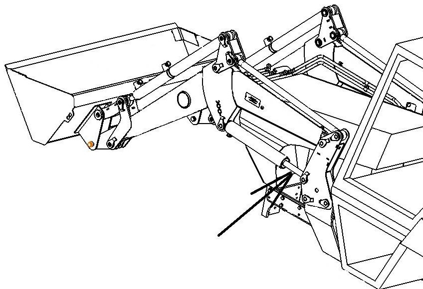
Рис.9А Установка ГЦ подъема.
