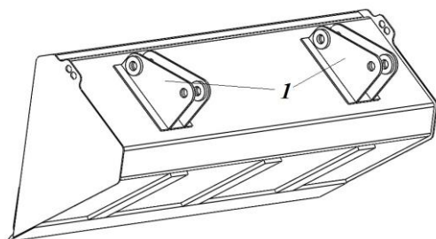
Рис.2 Ковш 0,22 м³ 1- кронштейн
