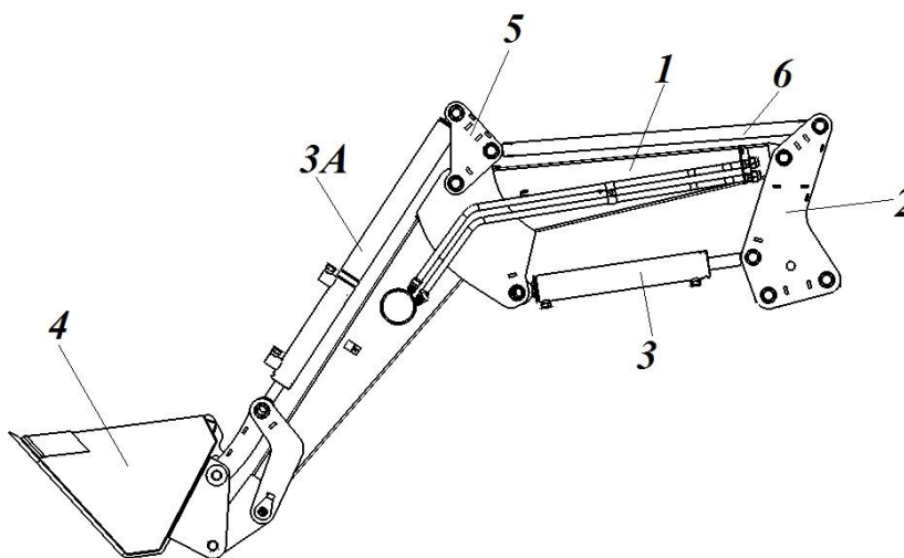
Рис.8 Подъемное устройство
