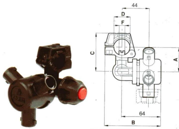
Соплодержатель трех позиционный-4064 247
