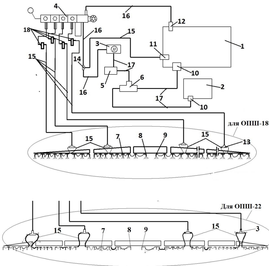
Рис.7 Схема работы и циркуляции жидкости
