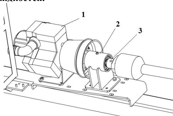
Рис.11 Насос мембранно-поршневой
