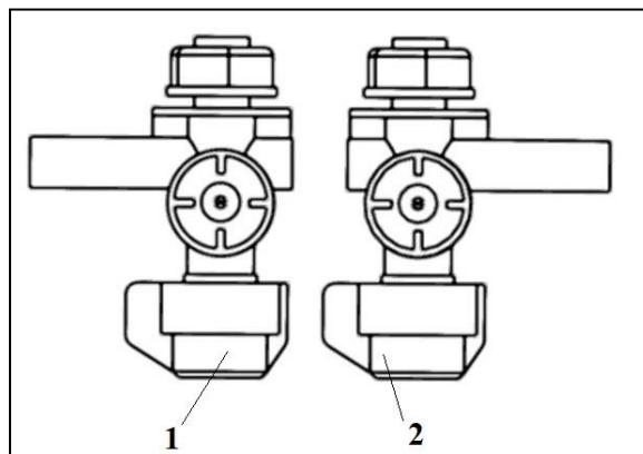
Рис.13 Распылитель щелевой проходной
