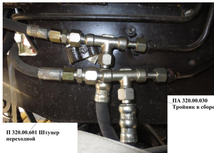
Рис.9 Подсоединение тройника ПА320.00.030 и штуцера переходного П320.00.601
