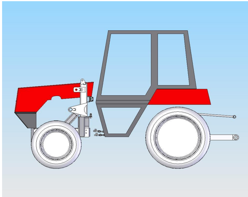
Рис.4. Навесное устройство 1-панель, 2- балка
