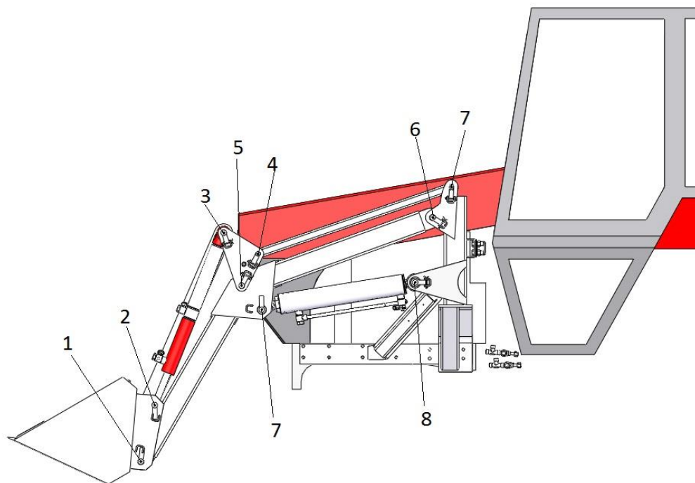
Рис.12. Схема смазки
