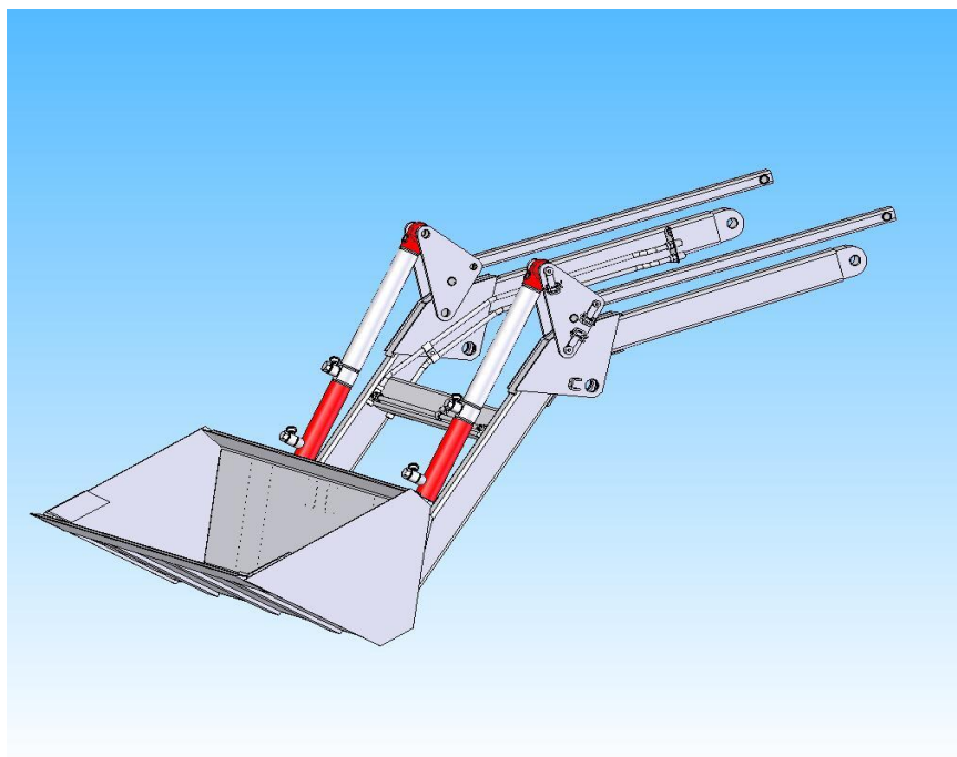
Рис.6 Подъемное устройство 1-рама подъема, 2-кронштейн, 3-ковш, 4- тяга, 5- гидроцилиндр
