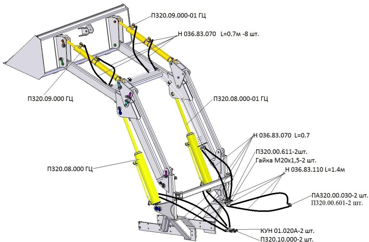
Рис.8 Схема подсоединения РВД
