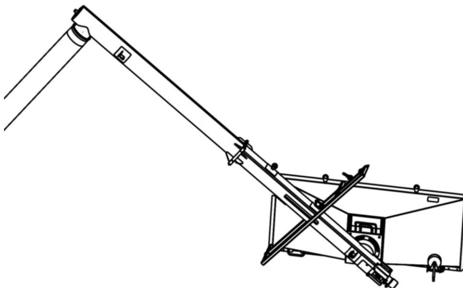
Рисунок 1 – Внешний вид загрузчика ЗСБ–30
