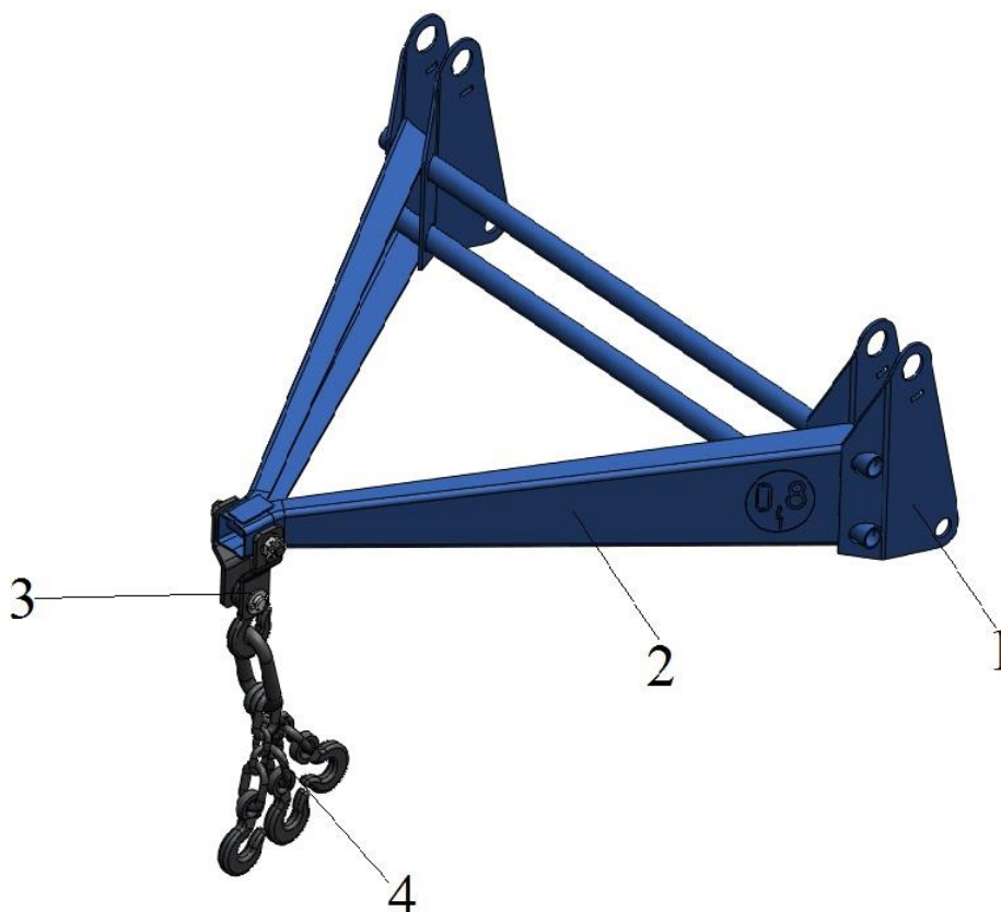
1- Кронштейн, 2-Рамка, 3-Крюк, 4-Расчалка
