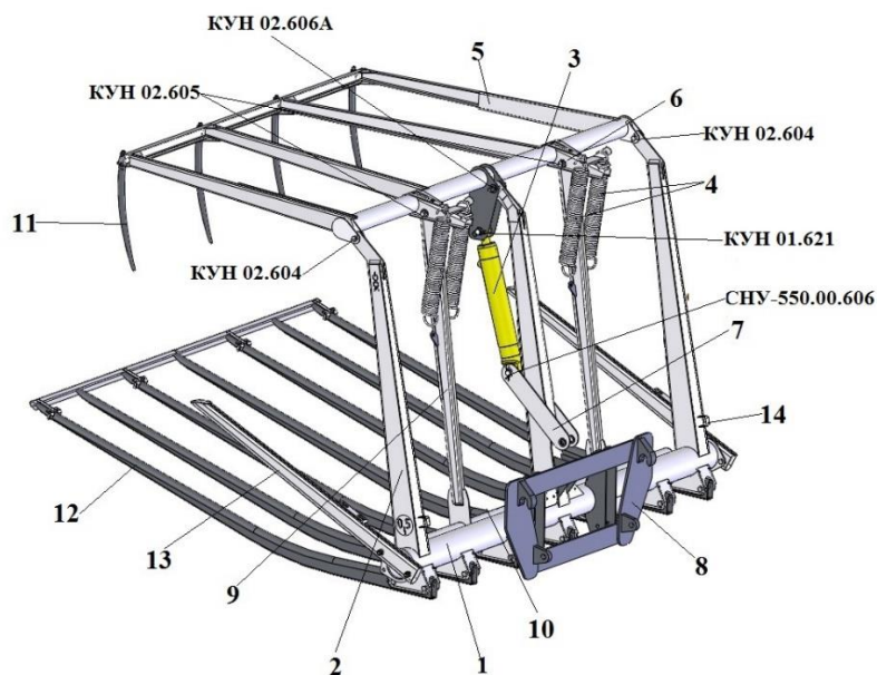
Рис.1 Решетка грабельная:
