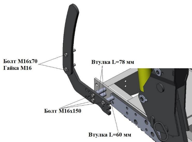
Рис.6 Ограждение
