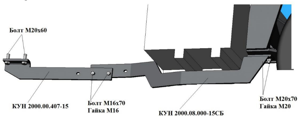
Рис.5 Тяга разгружающая
