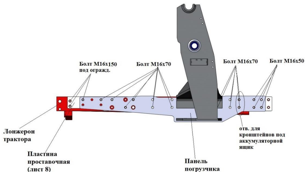
Рис.1 Панель навески
